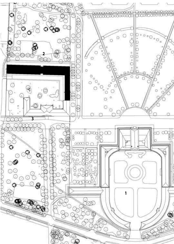
A most elkészült együttes viszonya a kastélyhoz
