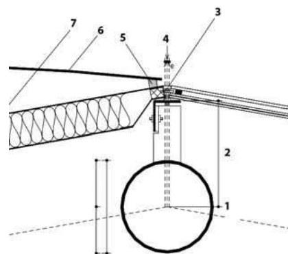
A héj eredetileg tervezett, de meg nem valósult csomópontja
