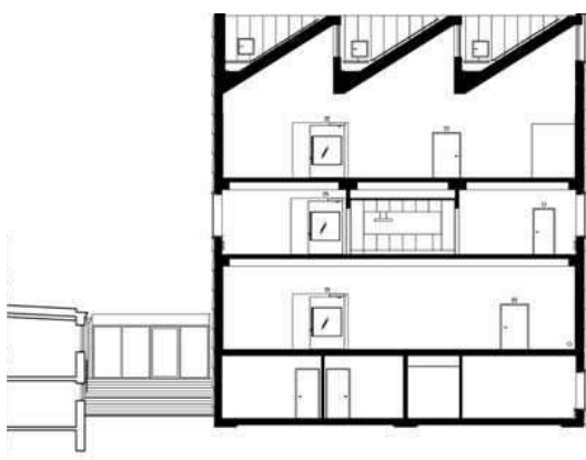
Perspektivikus és normál metszet
